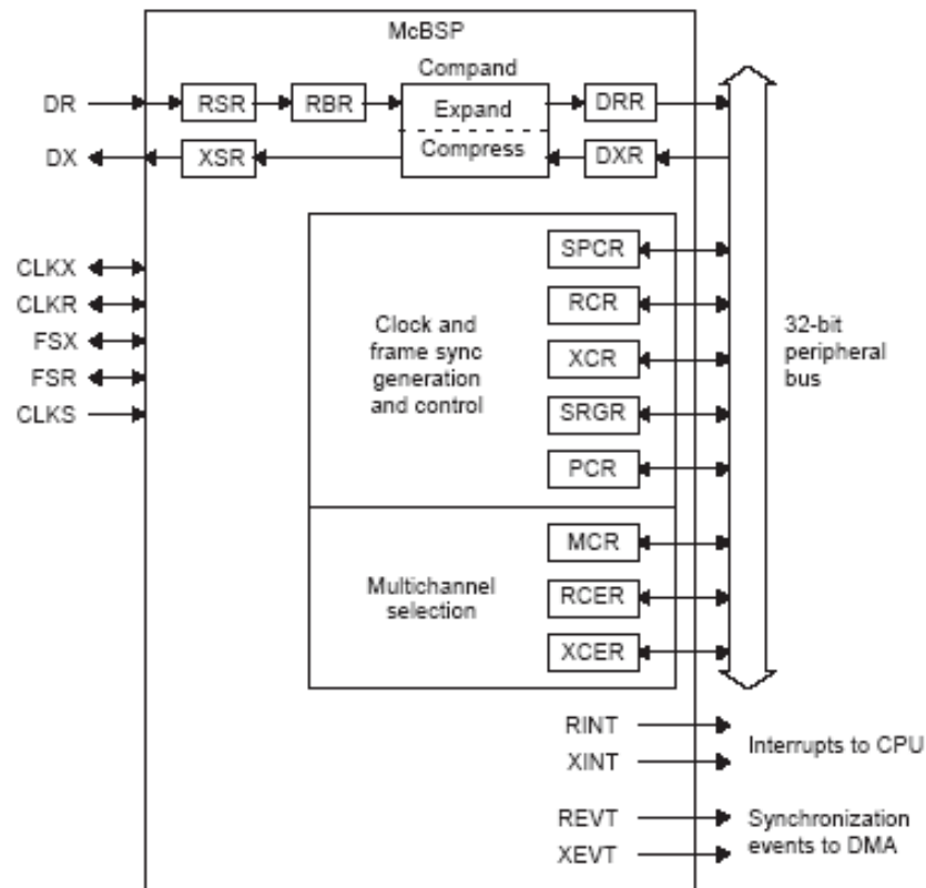
Figure.5.3 : Liaison série (McBSP)
