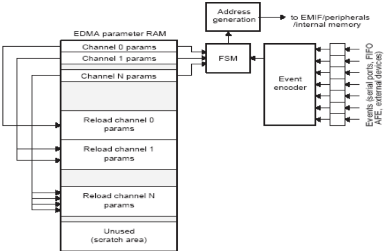
Figure.5.2 : Le contrôleur EDMA
