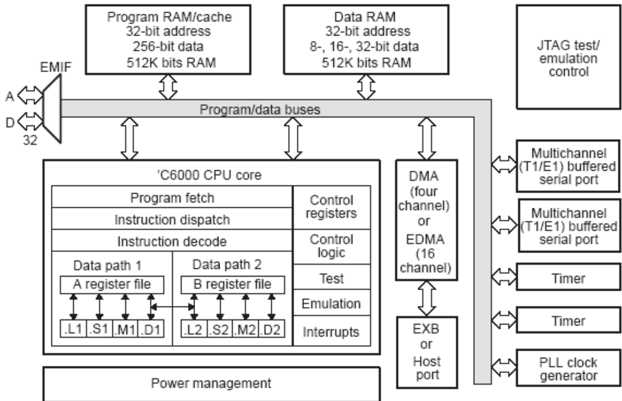
Figure 5.1 : Schéma fonctionnel du TMS320C67x
