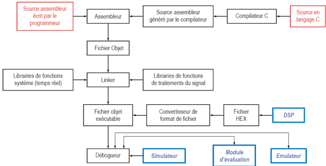
Figure 4.4 : Organigramme d'un système de développement de logiciel pour DSP
